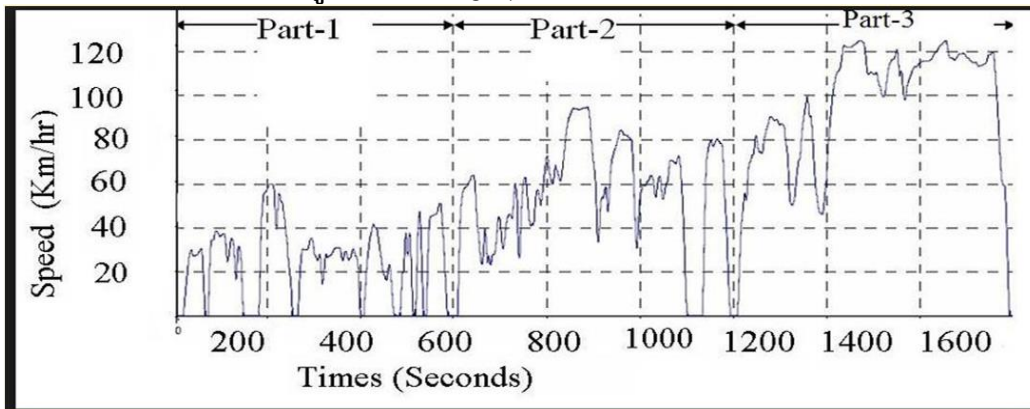
รูปที่ 6 Driving Cycle ตาม WMTTC, stage 2
