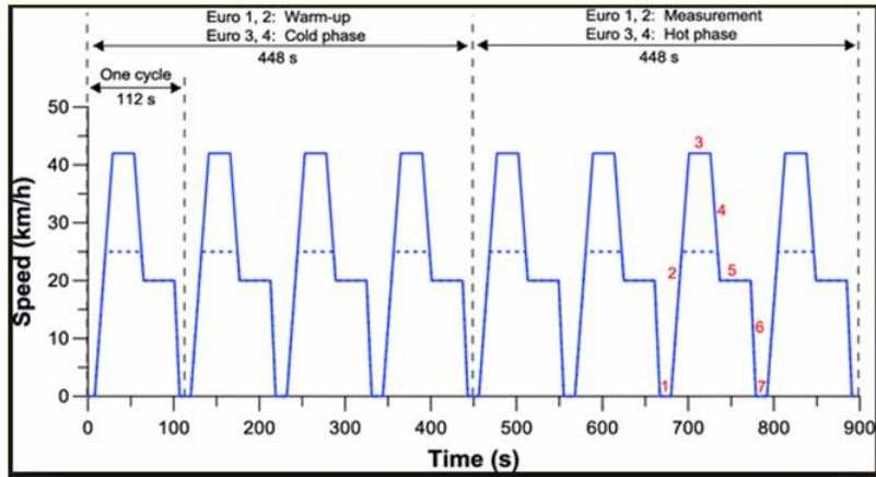
รูปที่ 5 Driving Cycle ตาม ECE R47
