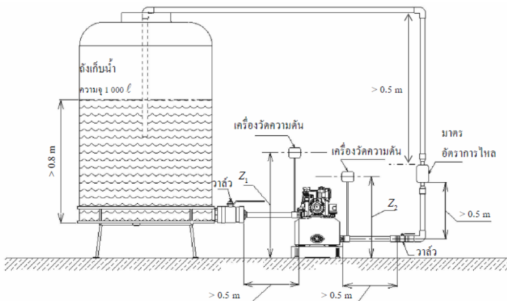
รูปที่ 3 การจัดวางเครื่องสูบน้ำไฟฟ้าชนิดอัตโนมัติ
