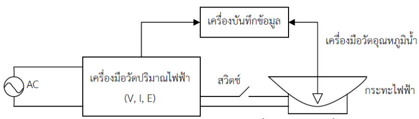
รูปที่ 3 แผนผังการติดตั้งกระทะไฟฟ้าและเครื่องมือวัด
