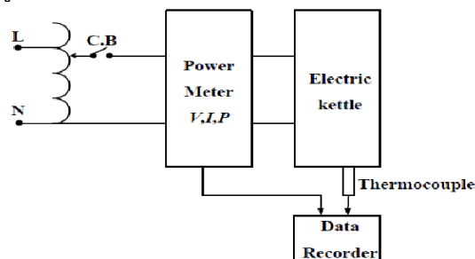
รูปที่ 3 รูปการต่อวงจรหาค่าประสิทธิภาพกาต้มน้ำไฟฟ้า
